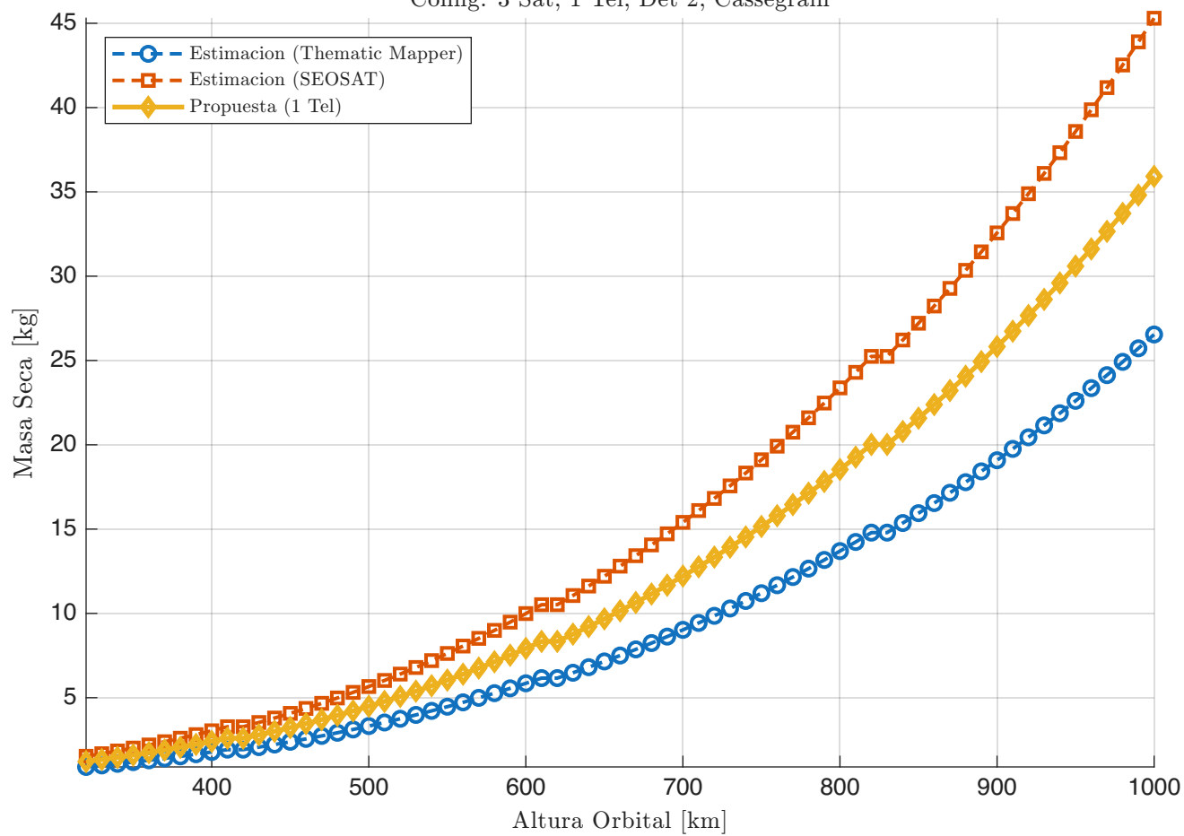
Comparativa de Masa Seca vs. Altura Config: 3 Sat, 1 Tel, Det 2, Cassegrain
